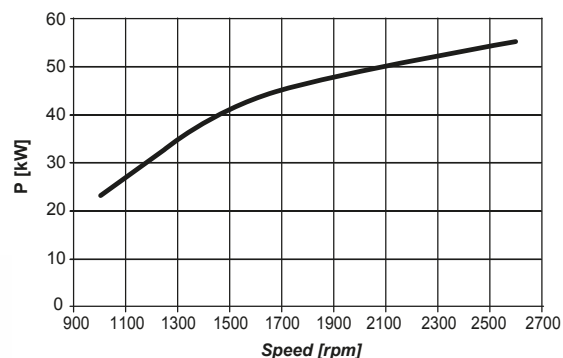
5.63D Deutz TD 2.9 L4 58 kW - 79 HP
